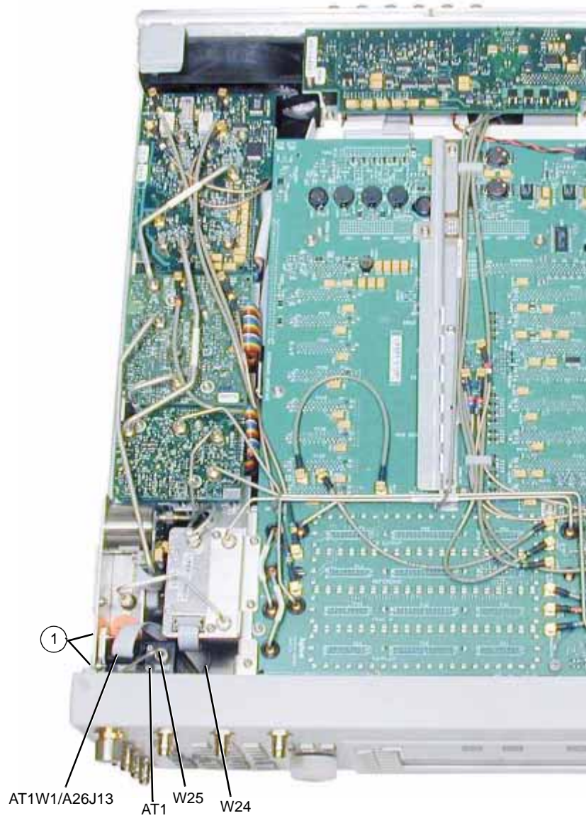
Figure 2-25 AT1 115 dB Attenuator (Option 1E1)
